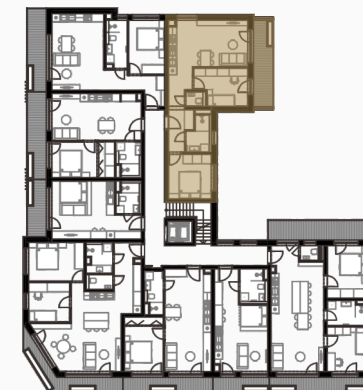
schéma pôdorysu
